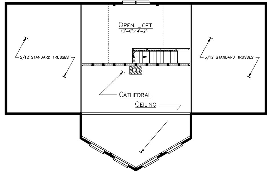
LOFT PLAN
